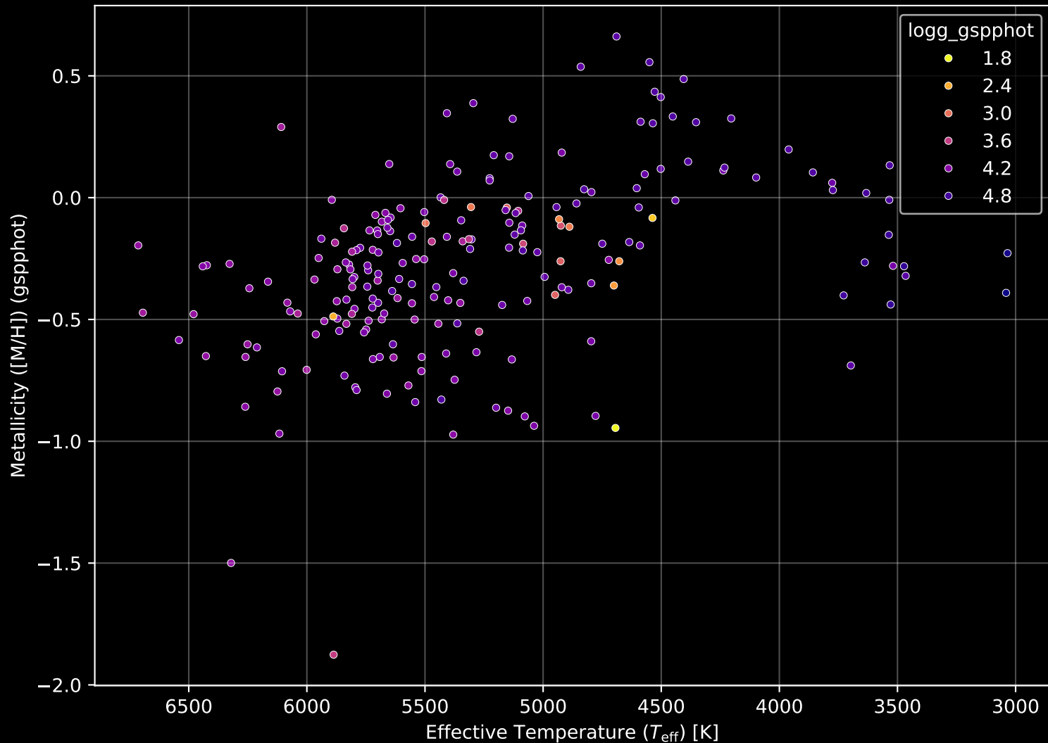
APOGEE DR17 Field: [126-55-O] Stellar Population Parameters (n= 216)
